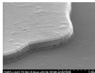
Réalisation de super-condensateur par RIE nano du CDC
