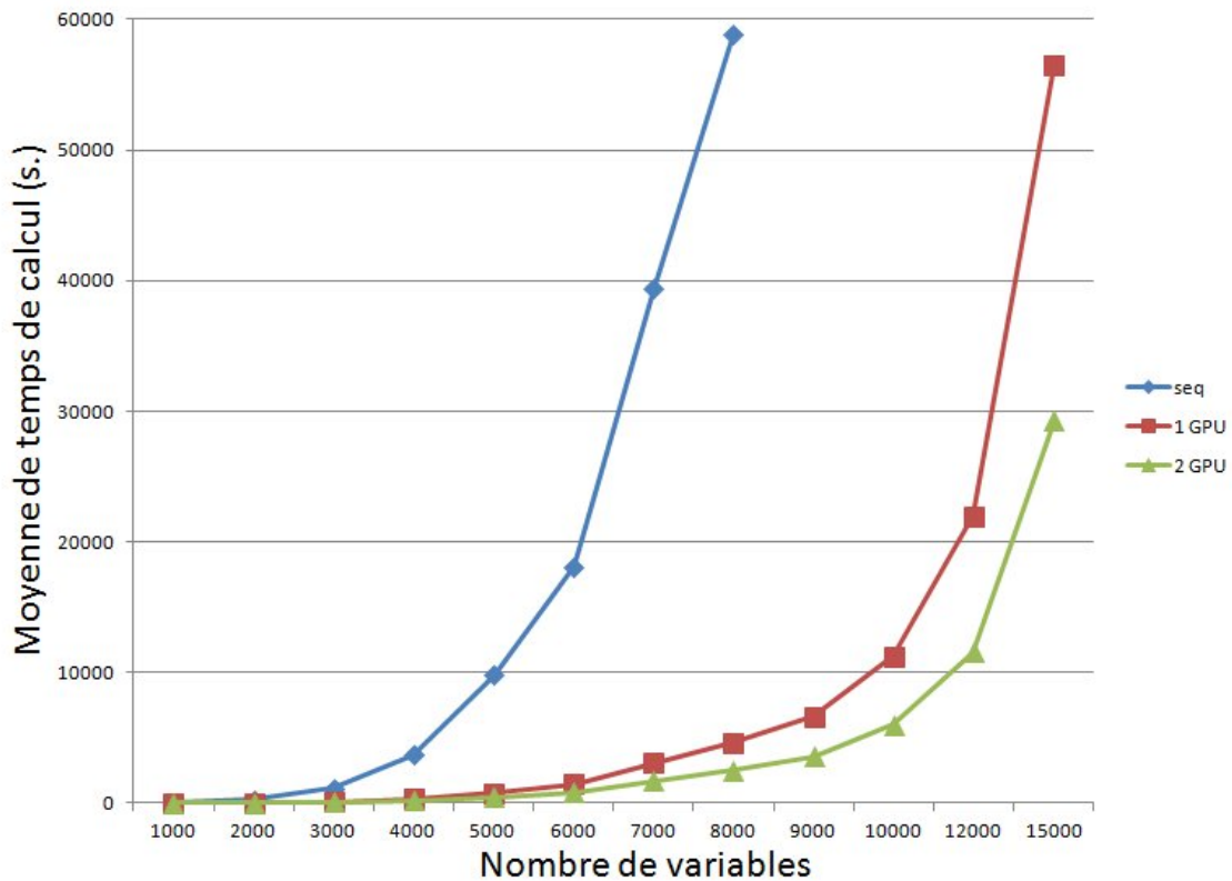
FIGURE VI.6 – Temps d’exécution de l’algorithme du Simplexe sur un CPU et différents systèmes avec un GPU et deux GPUs (Nvidia Tesla C2050).
