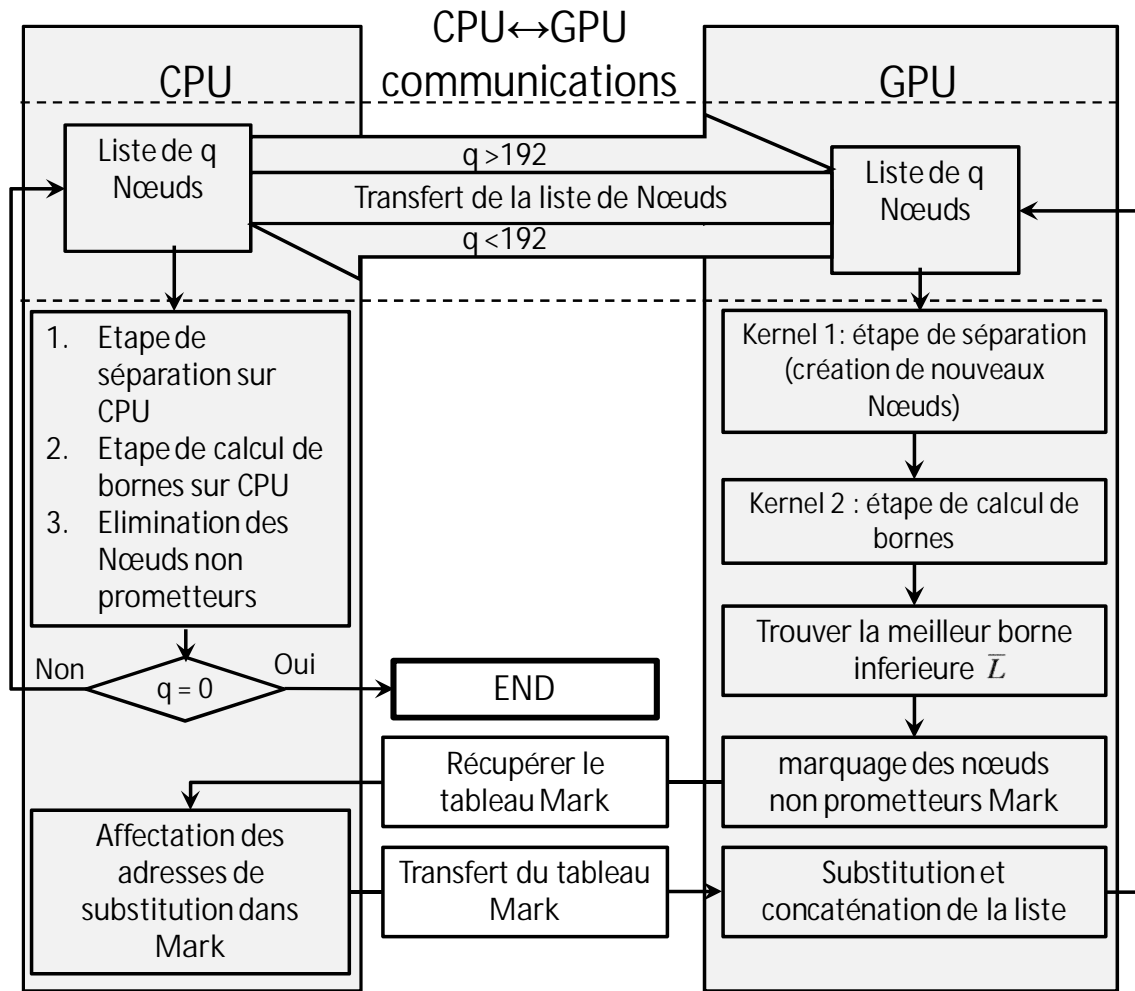
FIGURE V.2 – Algorithme de Branch and Bound sur système CPU-GPU.
