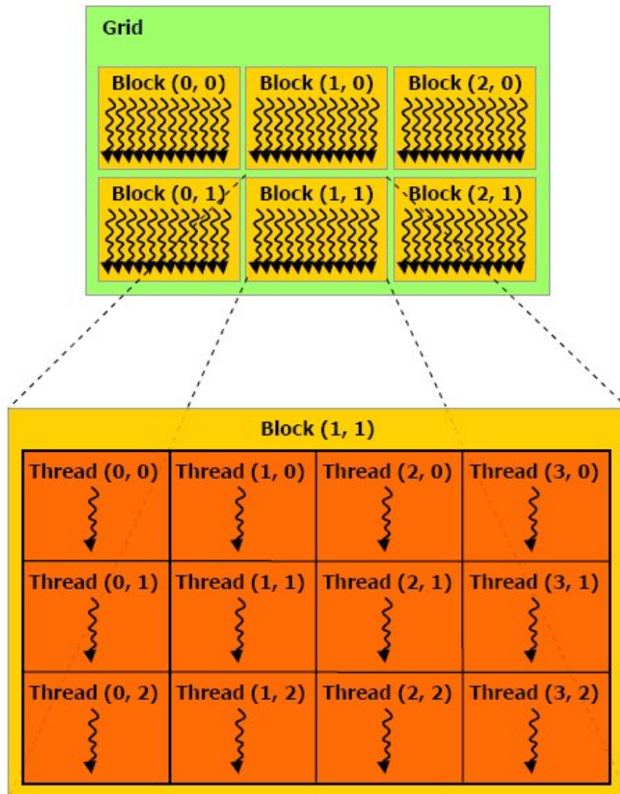
FIGURE IV.4 – Illustration d'une grille de threads (NVIDIA).
