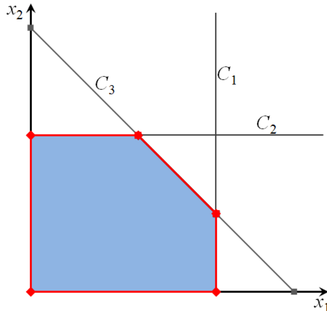
FIGURE VI.2 – Représentation géométrique du polytope pour un exemple avec n = 2 et m = 3 .
