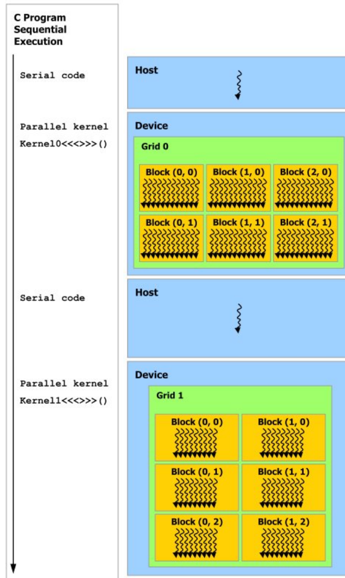
FIGURE IV.5 – Déroulement du programme sur CPU faisant intervenir le GPU (NVIDIA).
