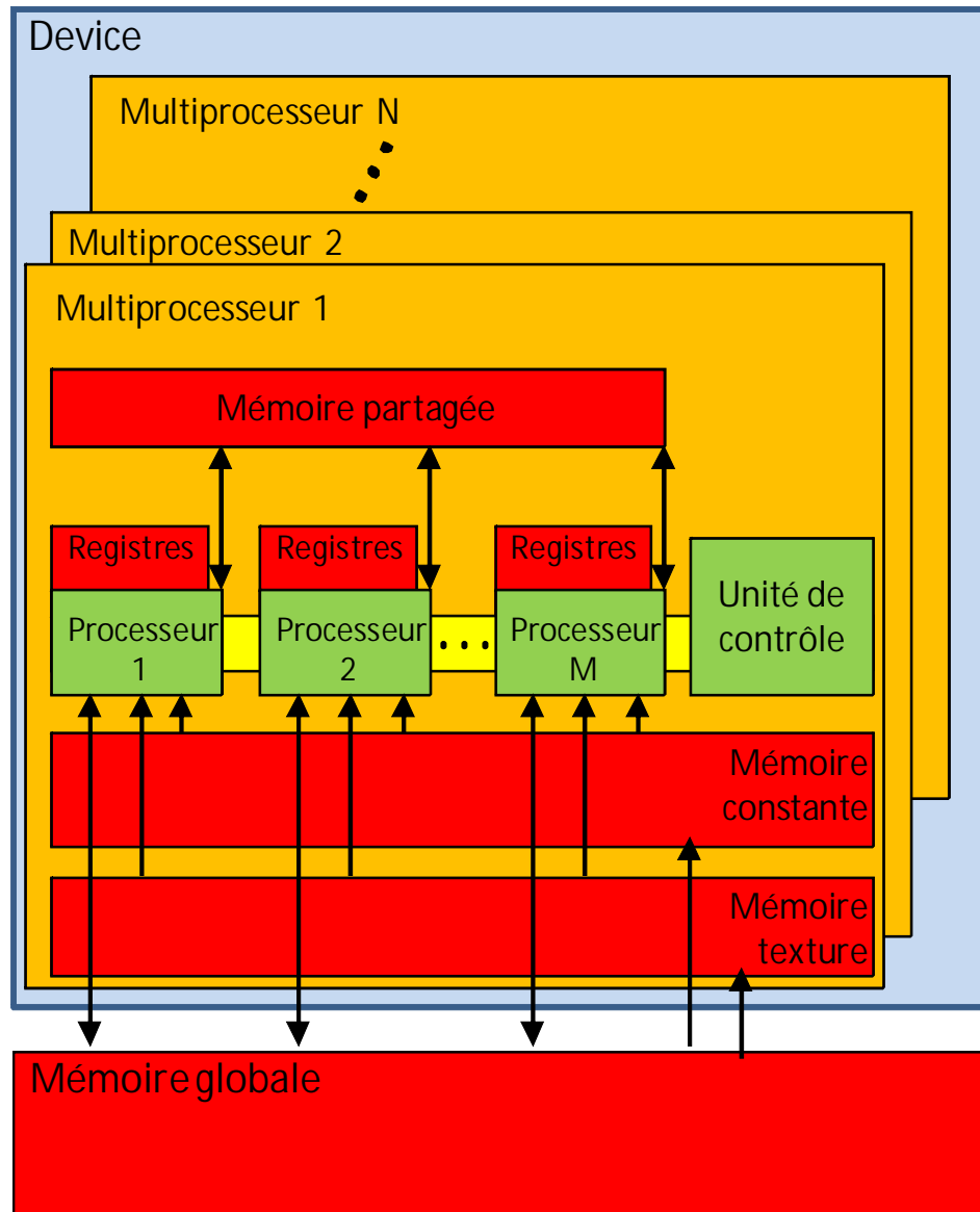
FIGURE IV.6 – Multiprocesseur SIMT avec mémoire partagée embarquée (NVIDIA).
