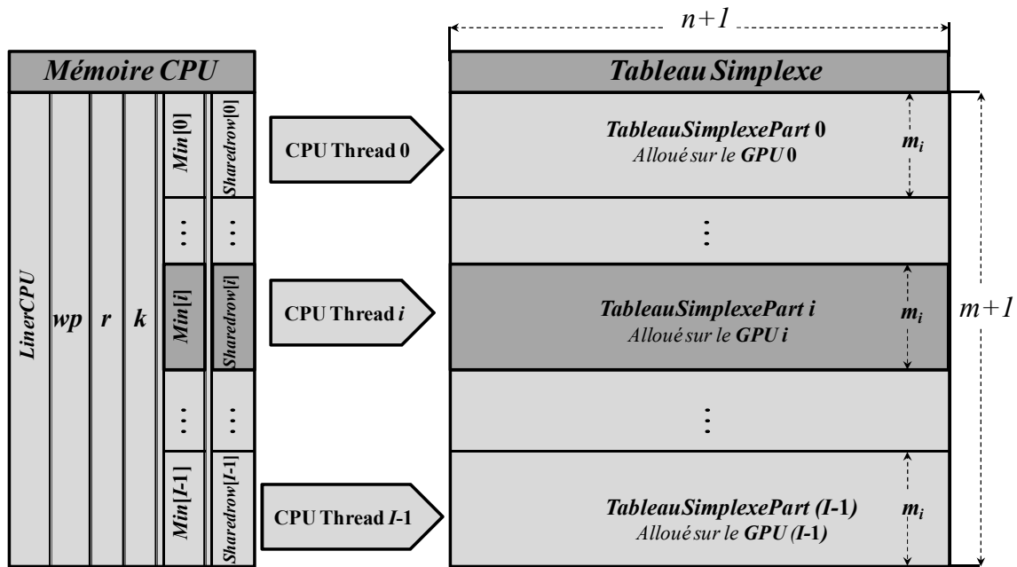
FIGURE VI.5 – Décomposition du TableauSimplexe et accès mémoire des threads CPU.
