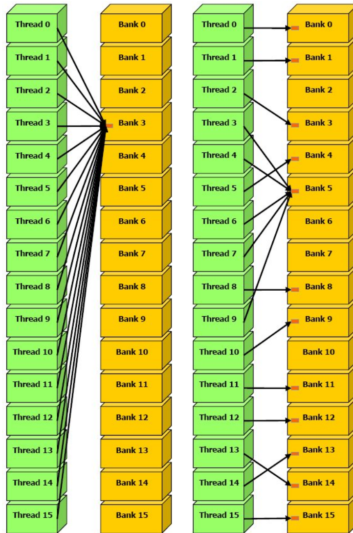
FIGURE IV.9 – Adressages à la mémoire partagée avec diffusion (NVIDIA).
