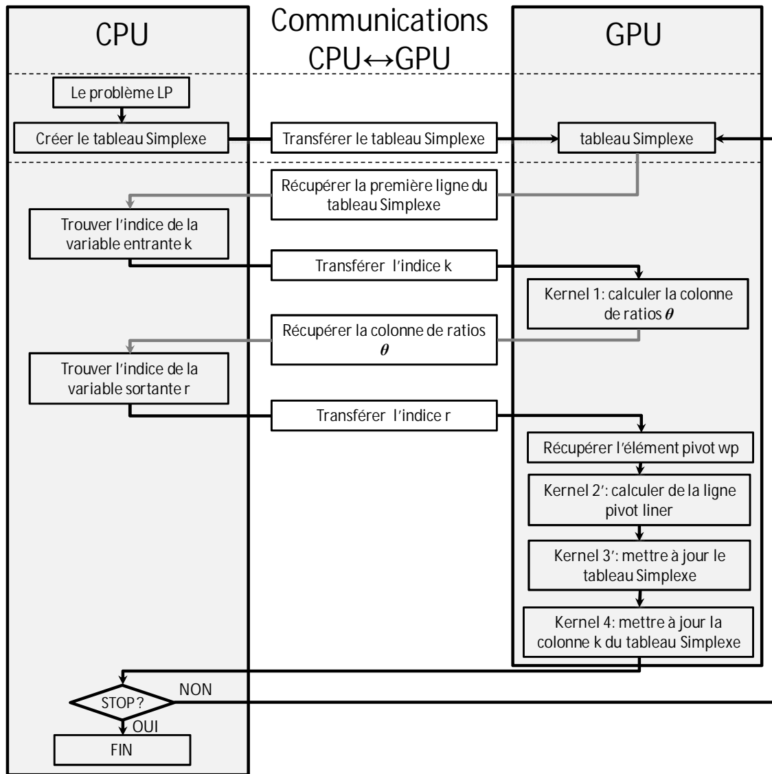
FIGURE VI.3 – Architecture globale de l’algorithme du Simplexe sur un système CPU-GPU.
