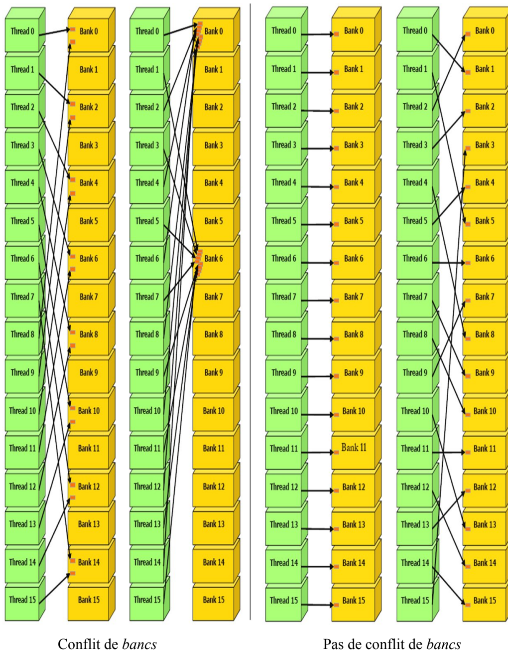
FIGURE IV.8 – Adressages à la mémoire partagée avec et sans conflit de bancs (NVIDIA).
