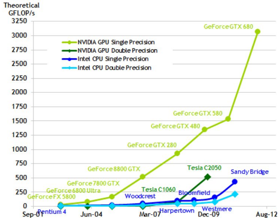
FIGURE IV.1 – Evolution des performances de calcul des CPUs et GPUs (NVIDIA).
