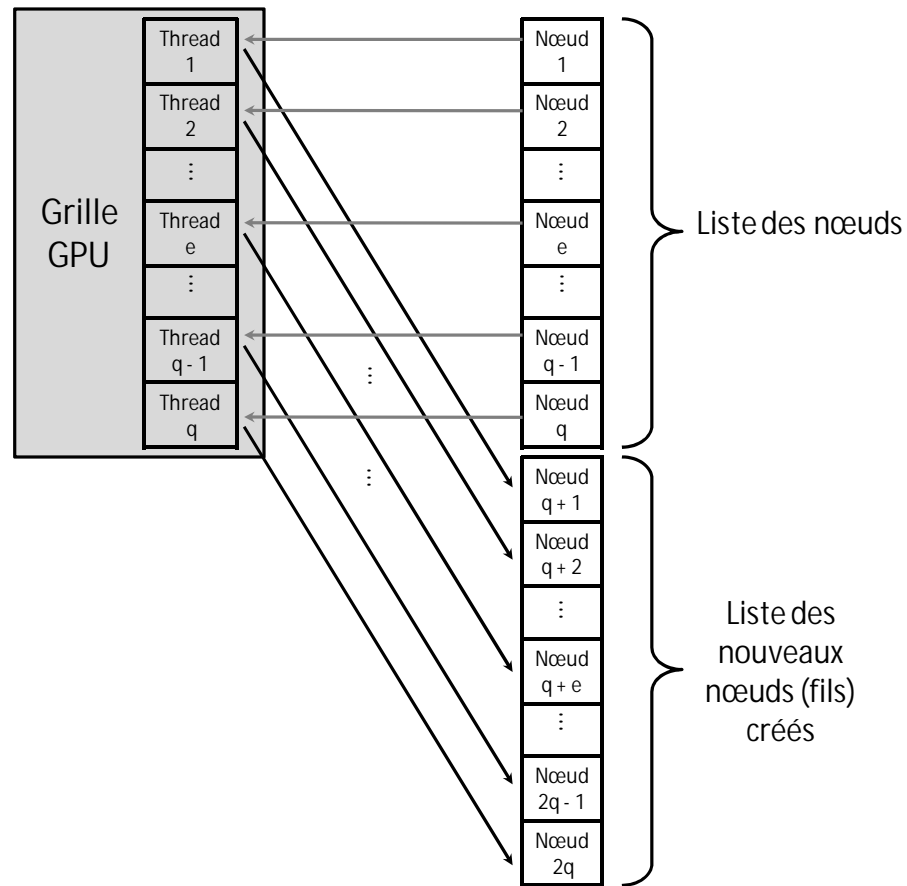
FIGURE V.3 – Création de nouveaux nœuds par la grille de threads sur GPU.
