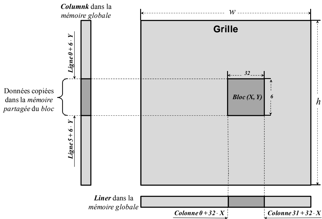
FIGURE VI.4 – Operations matricielles, gestion de mémoire dans le Kernel 3 '.
