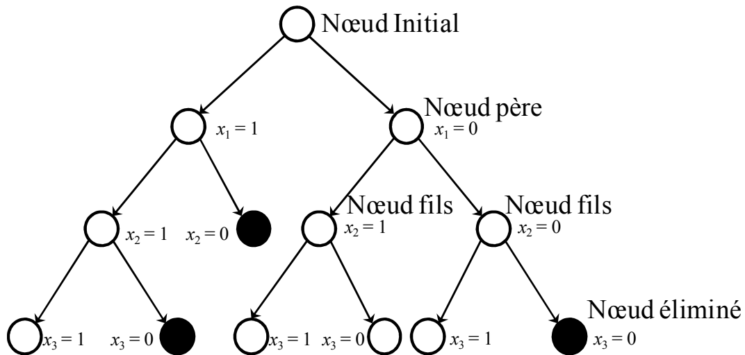
FIGURE II.1 Arbre engendré par décomposition d'un problème.
