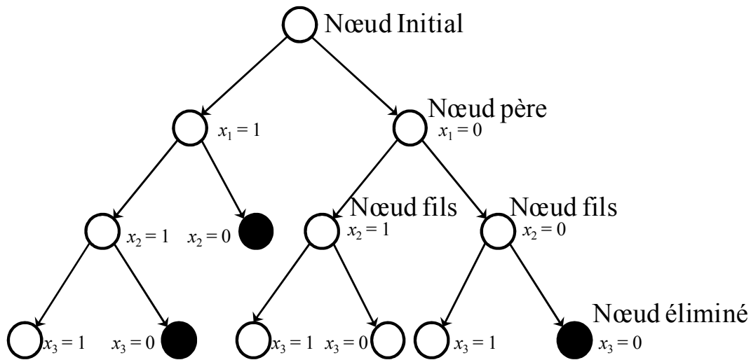
FIGURE V.2 – Arbre de décision
