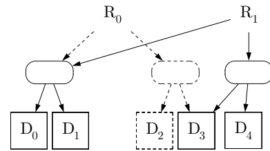
Figure 1. Encodage de plusieurs versions d'une séquence d'octets (fichier) sous forme d'un arbre [24]. Ici, une i-node est partagée entre les deux versions du fichier (dont les racines sont R_0 et R_1 ). Le bloc de données D_3 est également partagé.
